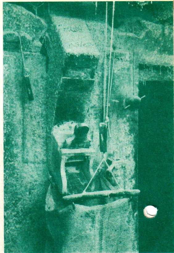
'Maalbak' met schuif op de Maxey Mill. Let op de zakophanging. Rechts naast de maalbak de licht (schroefdraad moer + losse sleutel). De knop rechtsboven dient voor het afstellen van het schoentje en is typisch Engels.
